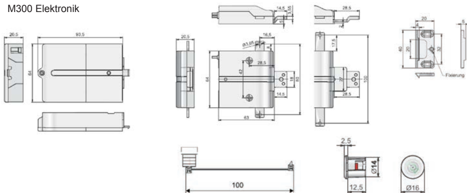
M300 Elektronik
